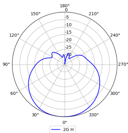
2.4GHz (水平)
