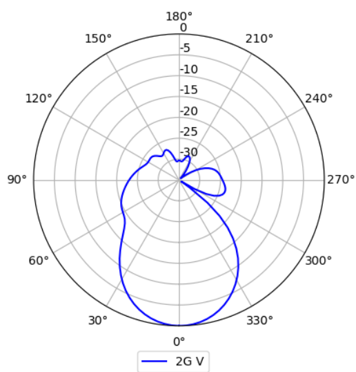
2.4GHz (垂直)
