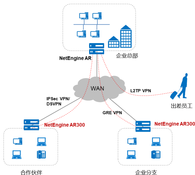
分支 VPN 组网场景
